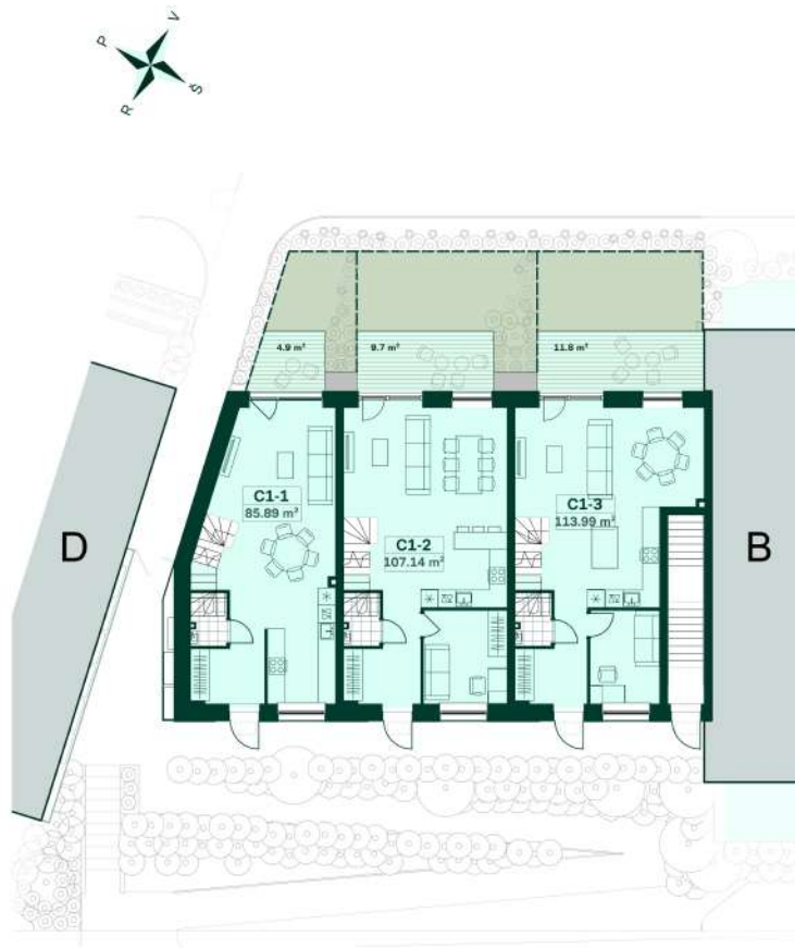
1 aukšto planas
