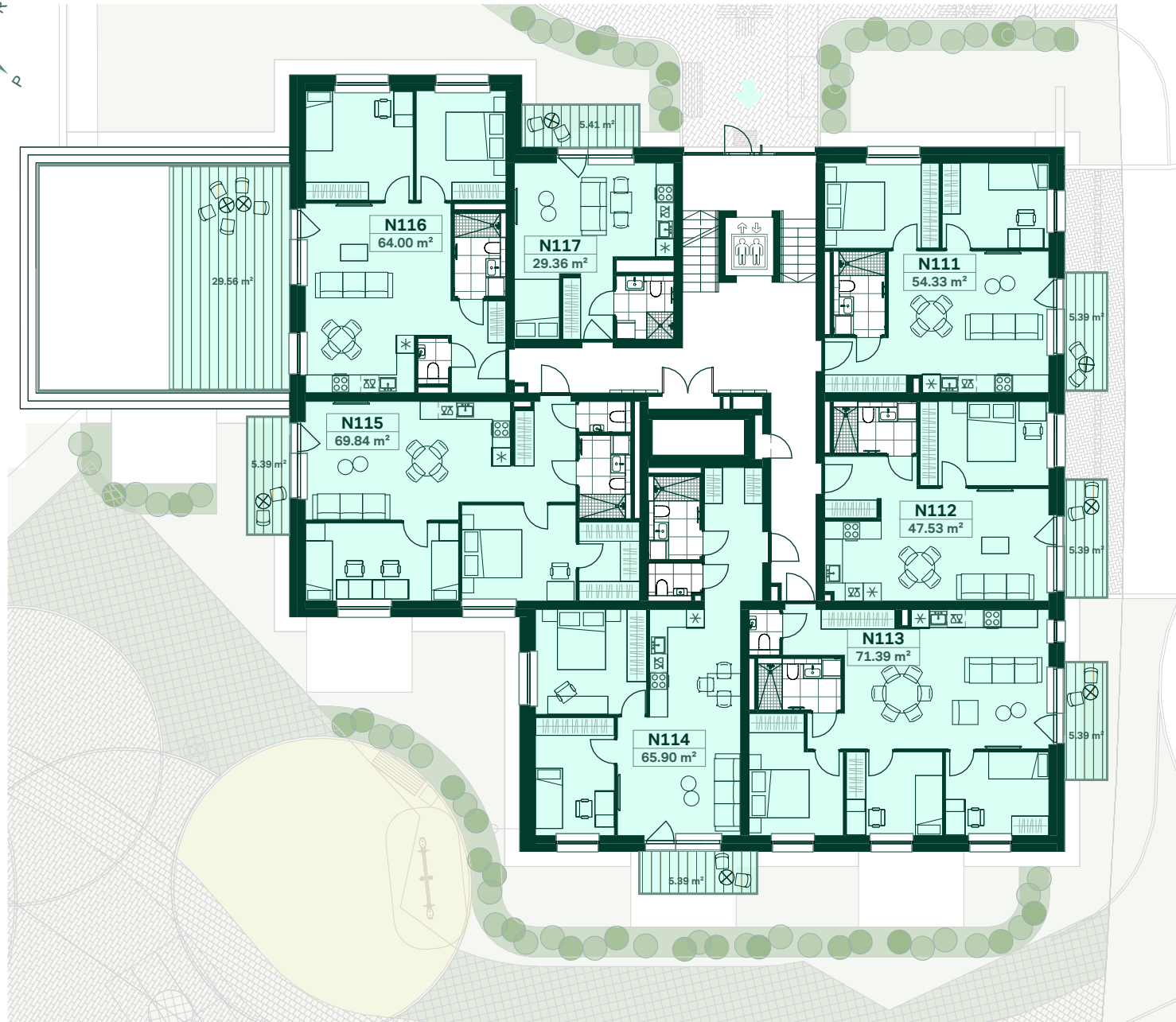
LAKE TOWN - N1 KORPUSAS, PIRMO AUKŠTO PLANAS Duisburgo g., Vilnius
